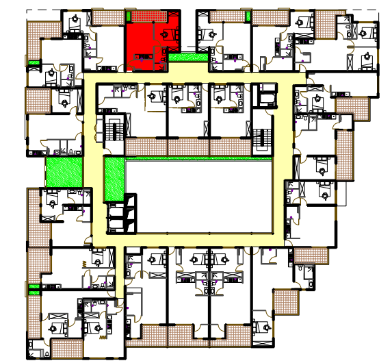
Plan du R+2 à R+6 (étage courant) sans échelle
