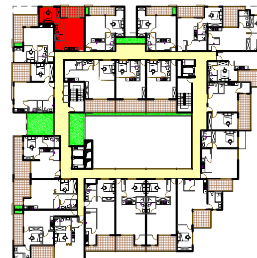
Plan du R+2 à R+6 (étage courant) sans échelle
