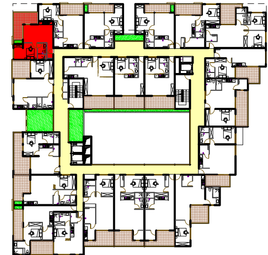
Plan du R+2 à R+6 (étage écarté) sans échelle
